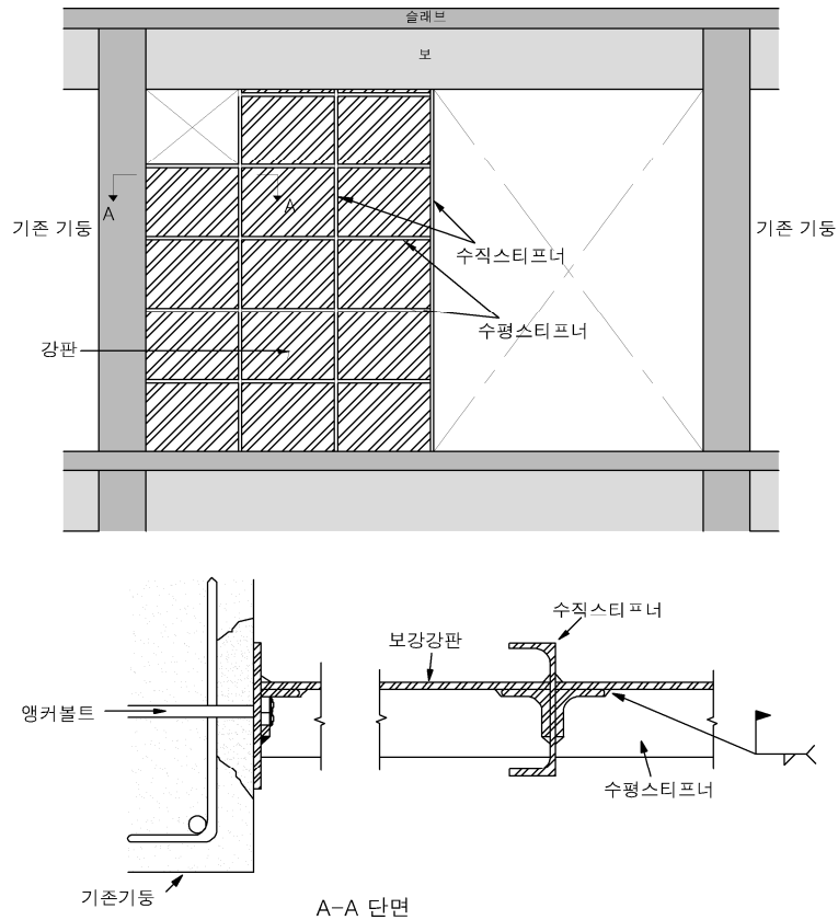
[그림 11-10] 강판 채움벽 신설
