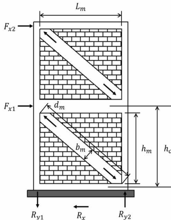
[그림 6-1] 등가스트럿 모델
