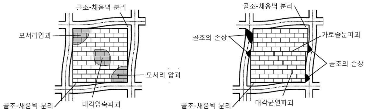
[해그림 6-6] 조적채움파괴모드 (Asteris, 2011)
