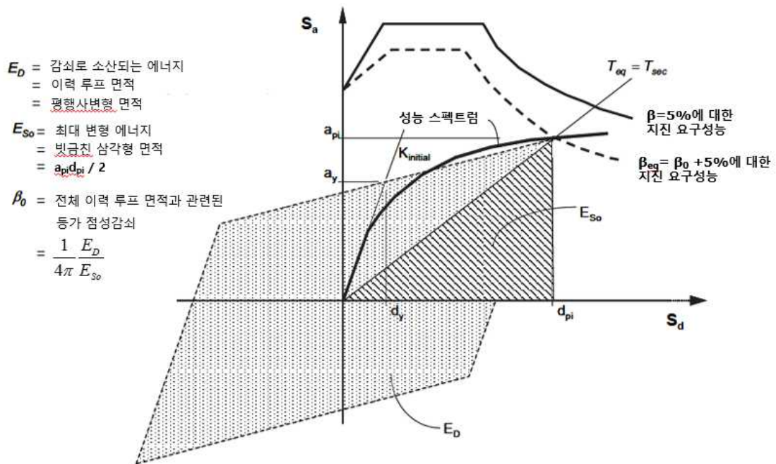
[해그림 4-7] 역량스펙트럼법
