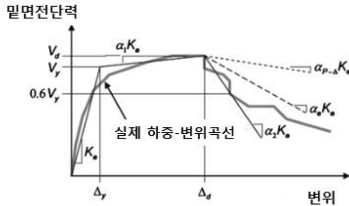
[해그림 4-8] 유효감성의 결정
