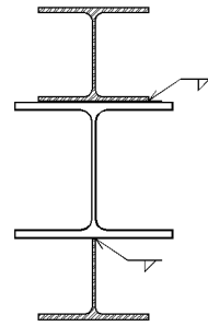
(b) H형강 보 상하부 형강 보강
