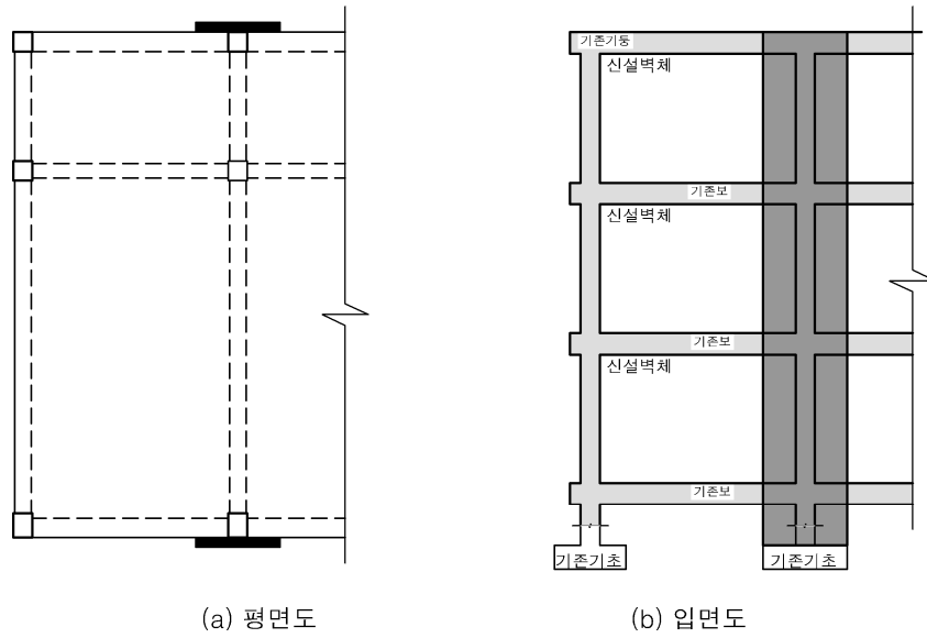
[그림 11-13] 프리캐스트 콘크리트벽 증설의 예
