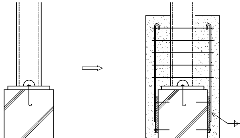
[그림 14-9] 주각부를 철근콘크리트로 감싼 보강 사례
