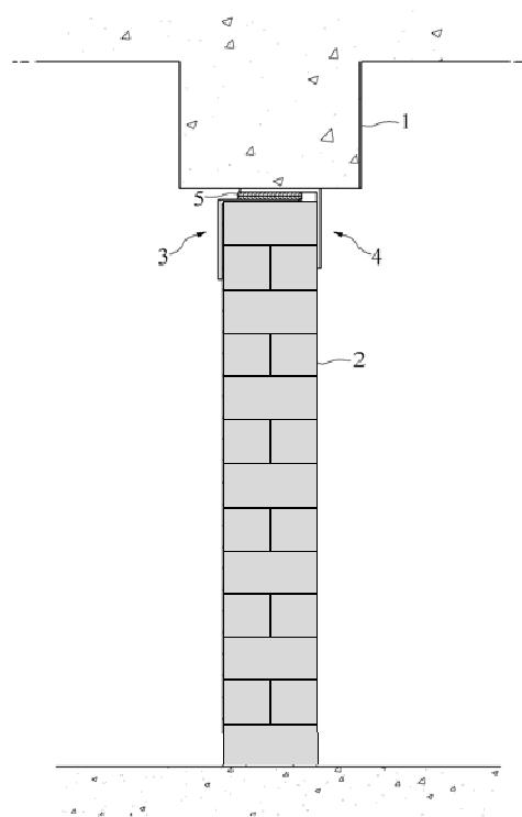
앵글과 덧댐판을 이용한 방법
