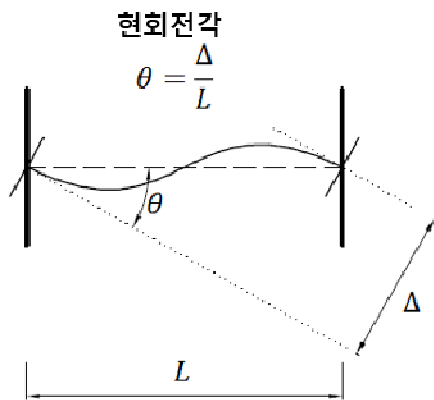
[그림 5-4] 전단벽 연결보의 현회전각
