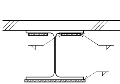
(a) H형강 보 상하부 강판 보강
