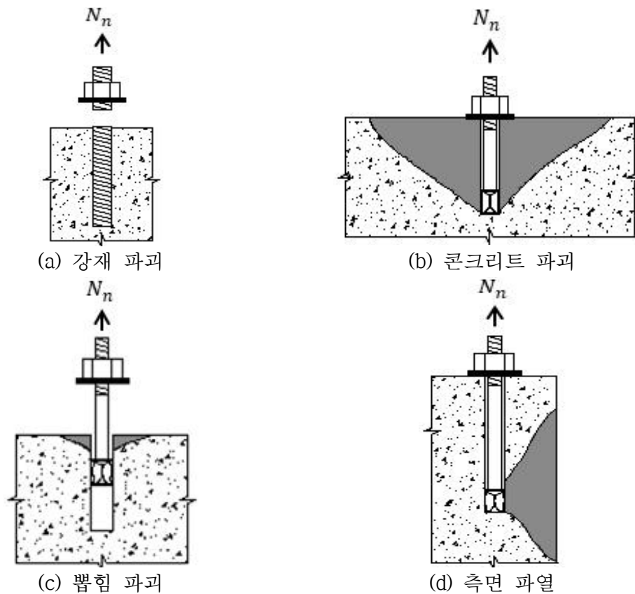
[그림 15-1] 인장에 의한 앵커의 파괴 유형
