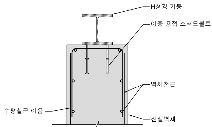
[그림 11-19] 채움벽 콘크리트 전단벽의 기둥-벽체 접합부 상세
