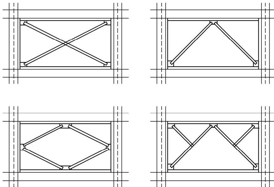
[그림 11-15] 중심가새 골조의 유형
