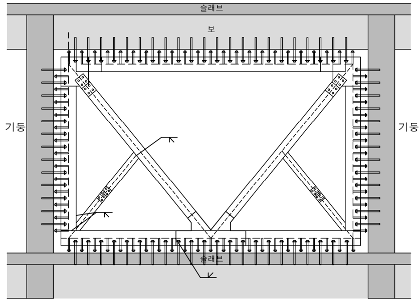
[해그림 11-4] 간접접합을 이용한 철골보강공법의 예
