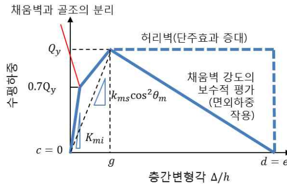
[해그림 6-7] 조적채움벽과 허리벽의 비선형정적절차 적용 모델
