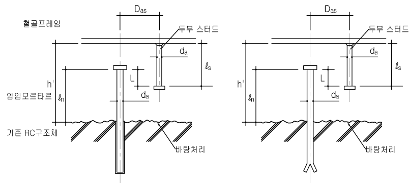
접착계 앵커
