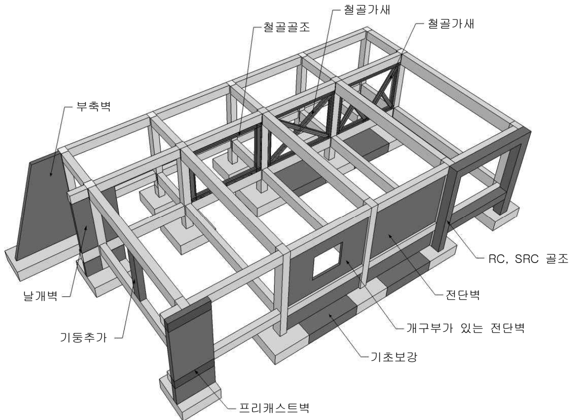
[그림 11-1] 주요 시스템보강공법의 종류
