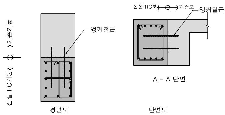
(a) RC와 기존 골조와의 접합상세
