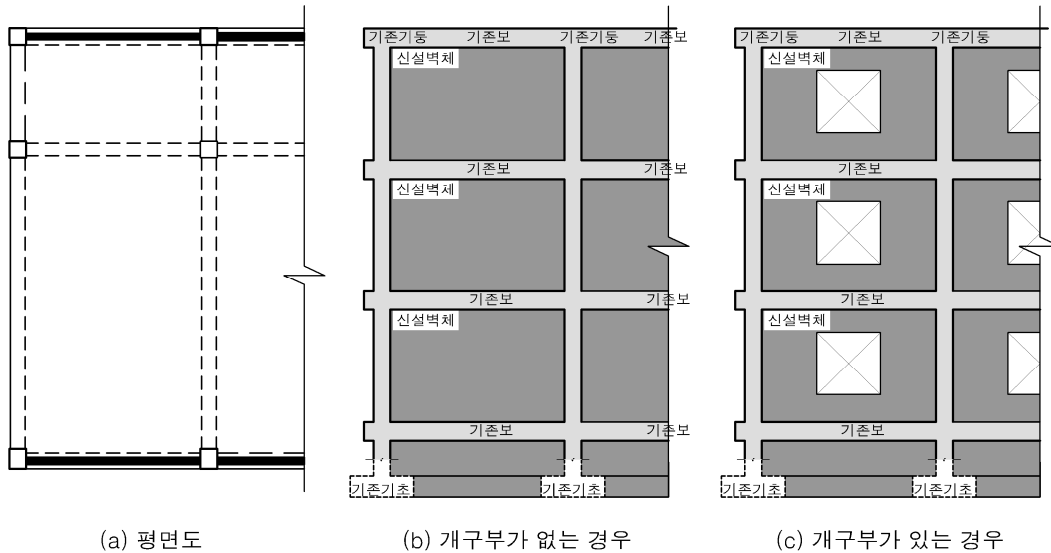
[그림 11-2] 콘크리트 채움벽 공법
