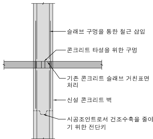
[그림 11-11] 기둥과 내력벽 신설
