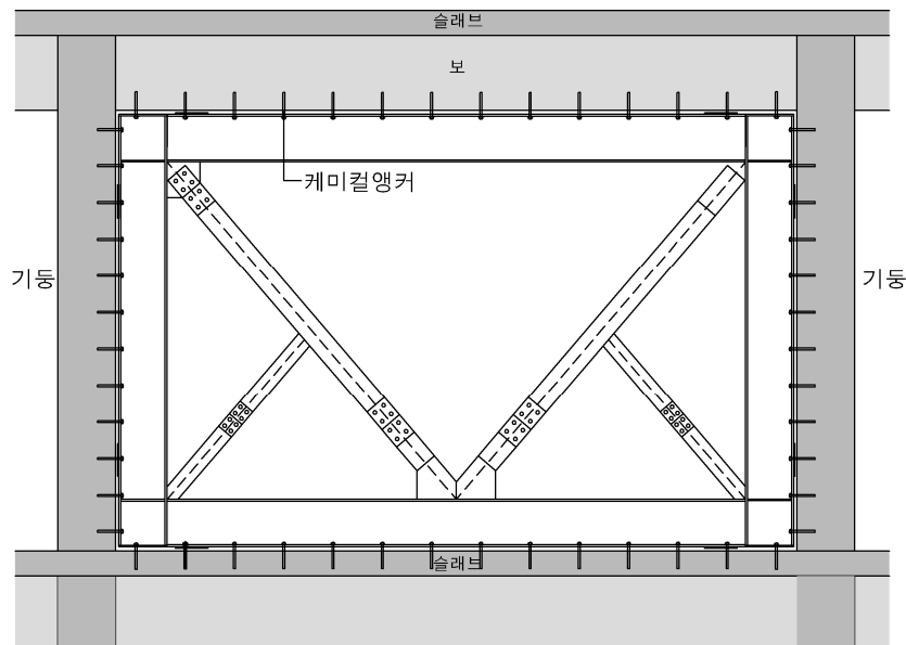
[해그림 11-3] 직접접합을 이용한 철골보강공법의 예
