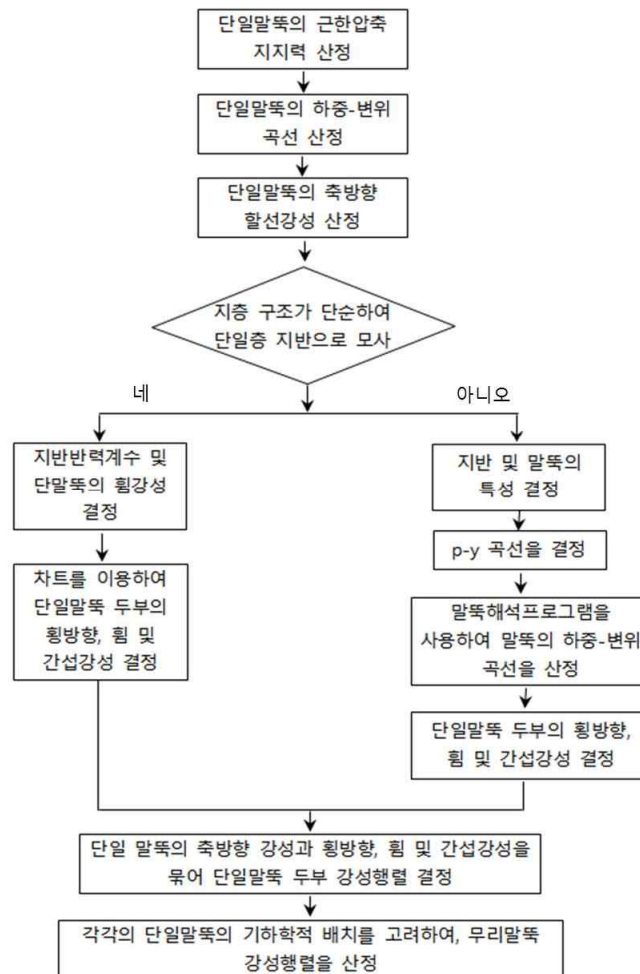
[해그림 8-3] 말뚝기초를 스프링으로 모델링하는 과정
