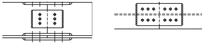
(a) 볼트접합 이음판 용접보강
