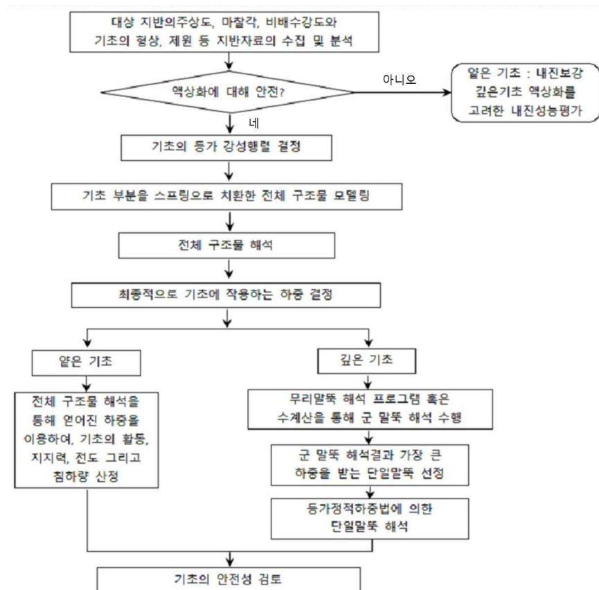
[해그림 8-1] 기초의 내진성능평가 절차
