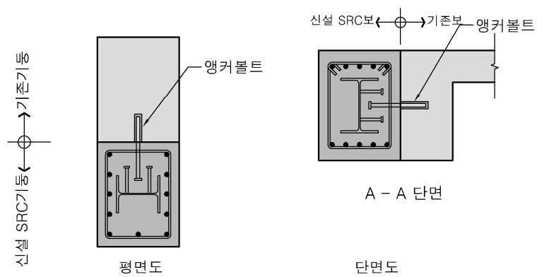
(b) SRC와 기존 골조와의 접합상세
