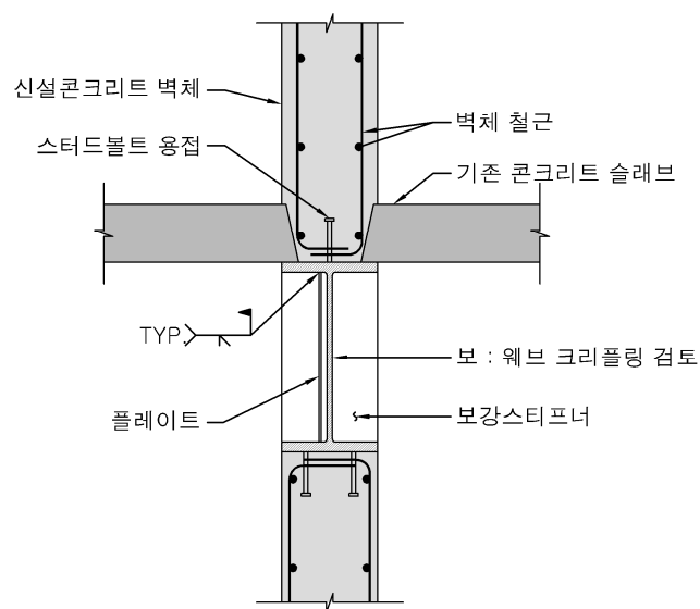
[그림 11-18] 채움벽 신설 콘크리트 전단벽의 보-벽체 접합부 상세
