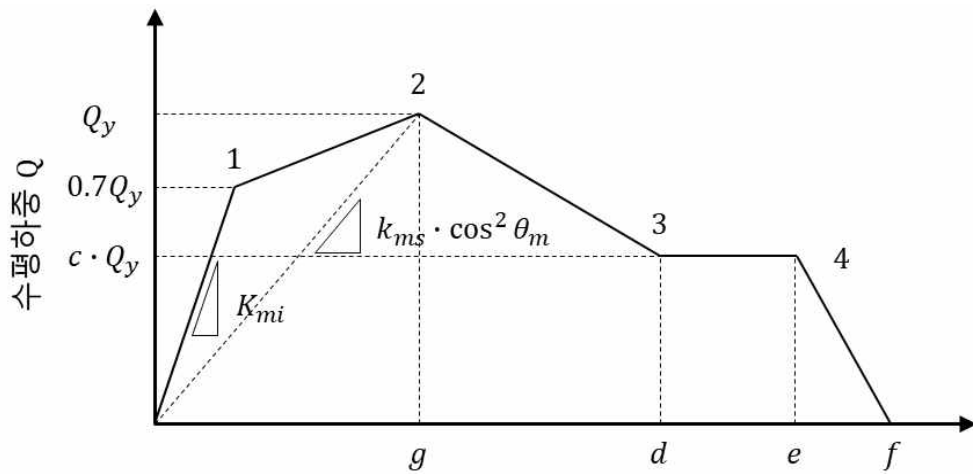
층간변형각 \Delta/h
