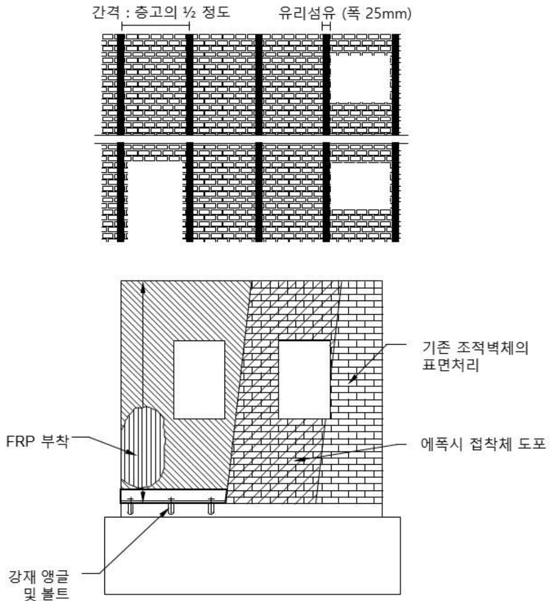
[그림 13-1] 섬유보강재 보강
