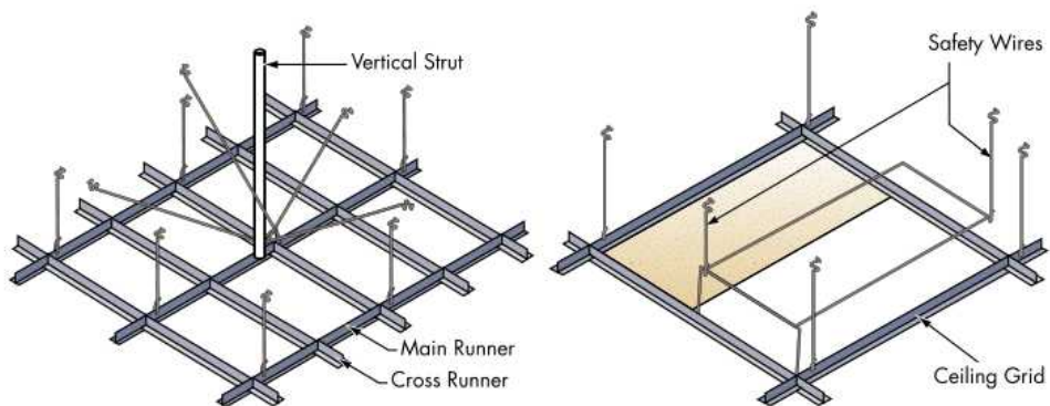
[해그림 17-5] 천장재의 지진 상세
