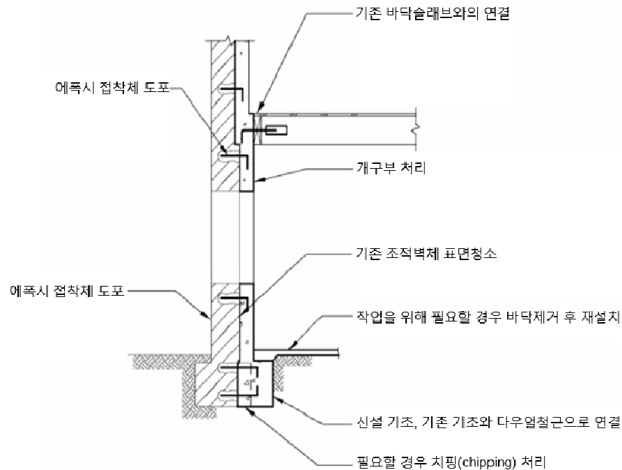
[그림 13-2] 조적채움벽체의 콘크리트/ 슷크리트 보강
