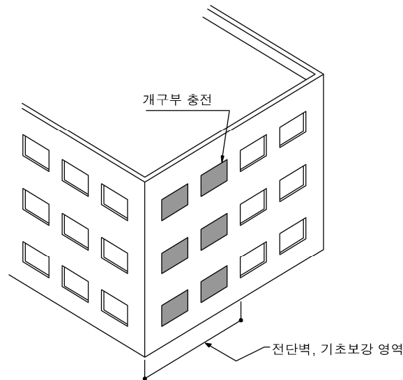
[그림 11-12] 개구부 충전을 통한 내진보강
