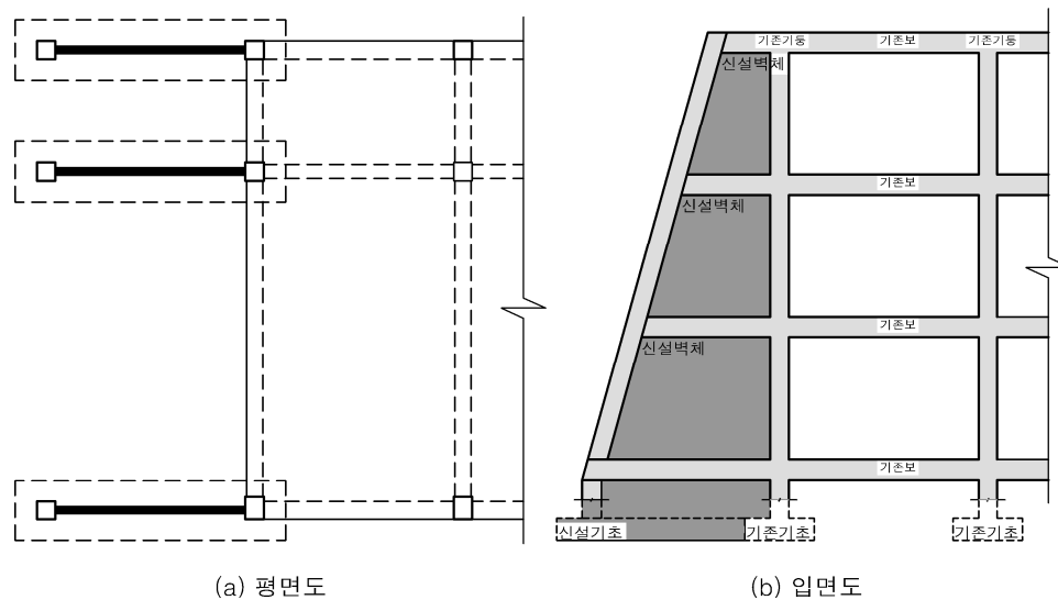
[그림 11-9] 부축벽 설치 공법
