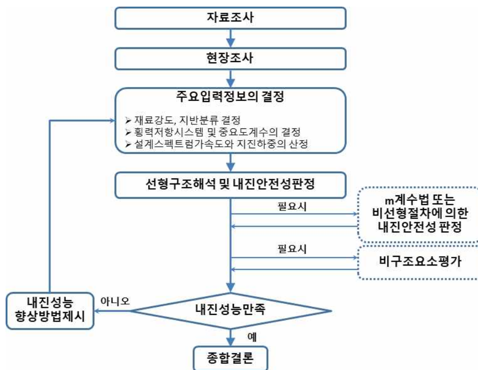
[그림 1-1] 내진성능평가절차
