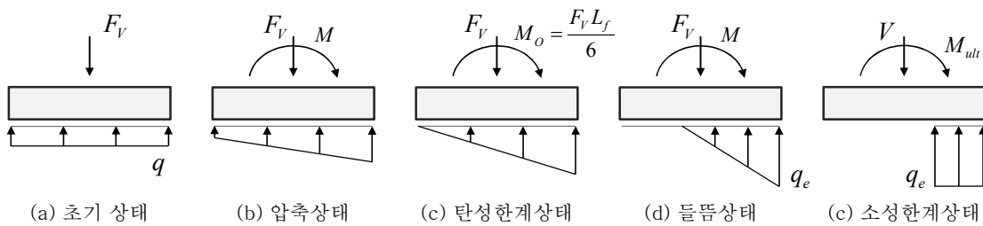
[해그림 8-4] 얇은기초에서 축력과 모멘트 조합에 따른 기초저면의 접지압 분포
