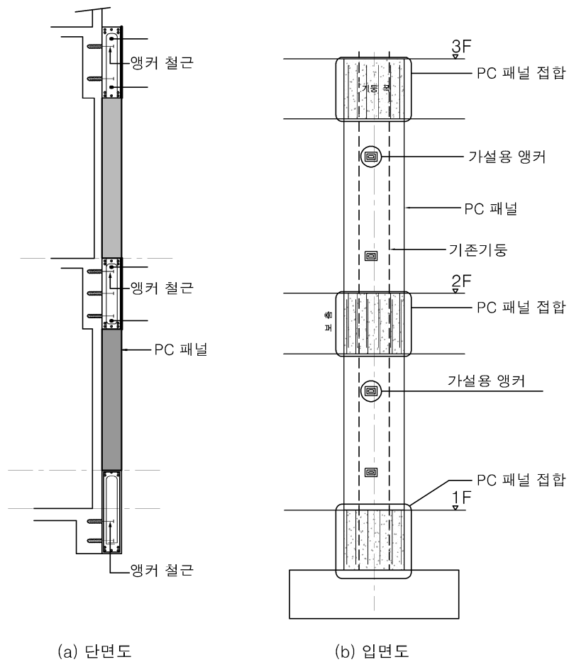
[그림 11-14] 프리캐스트 콘크리트벽의 연결상세 예
