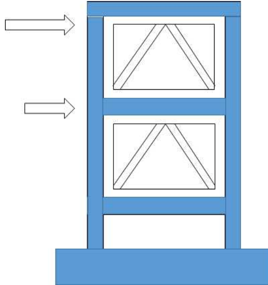
[해그림 18-1] 끼움가새를 사용하는 공법의 성능입증을 위한 실험체 구성의 예
