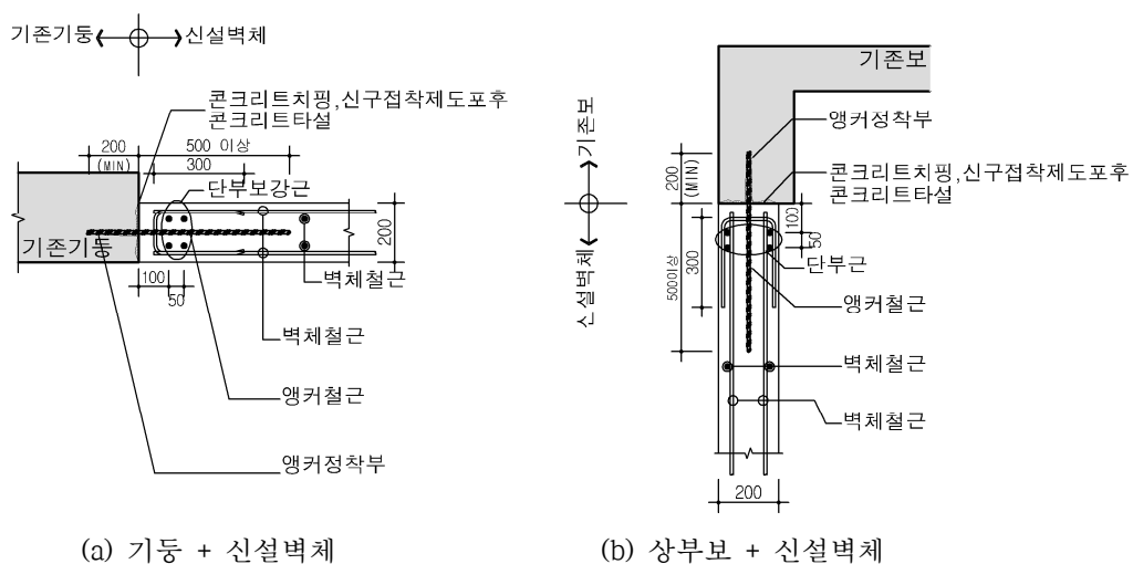
[해그림 11-2] 보 및 기둥과 전단벽의 연결 상세
