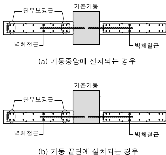
[그림 11-5] 기둥날개벽 증설 상세
