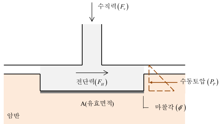
[해그림 8-5] 얕은기초에서 전단력에 대한 검토
