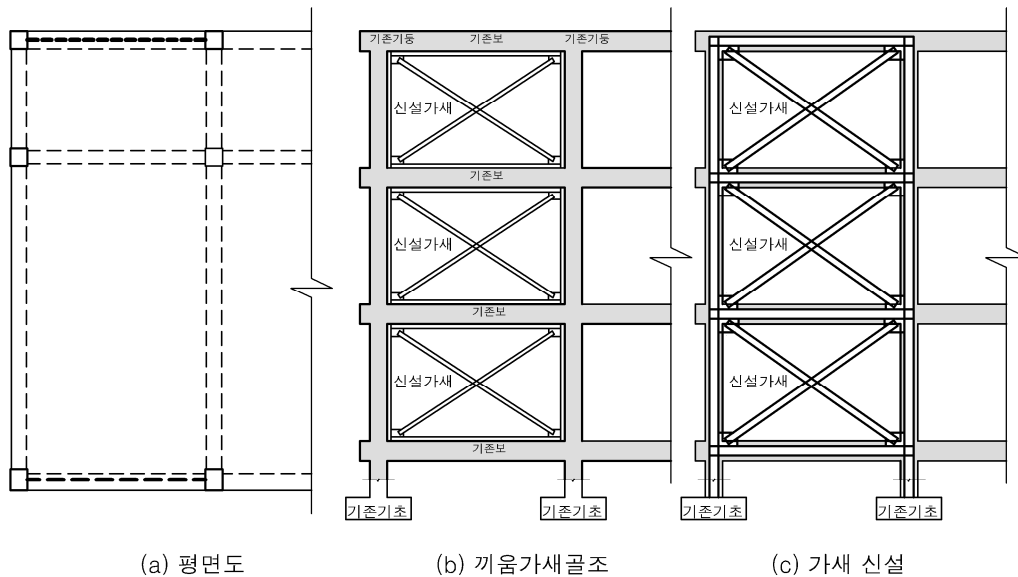
[그림 11-8] 끼움철골가새 및 철골가새 신설
