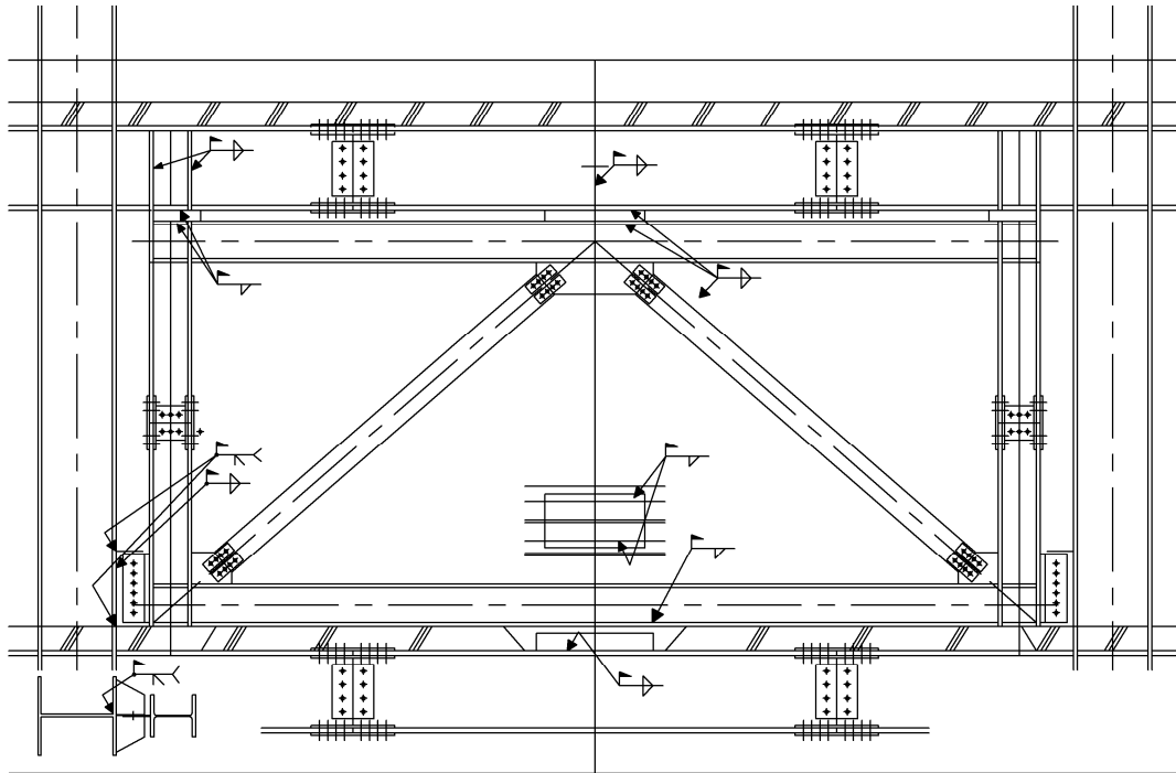
[그림 11-16] 철골 끼움골조의 신설
