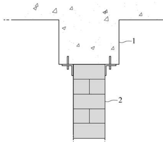
앵글과 철물을 사용한 방법
