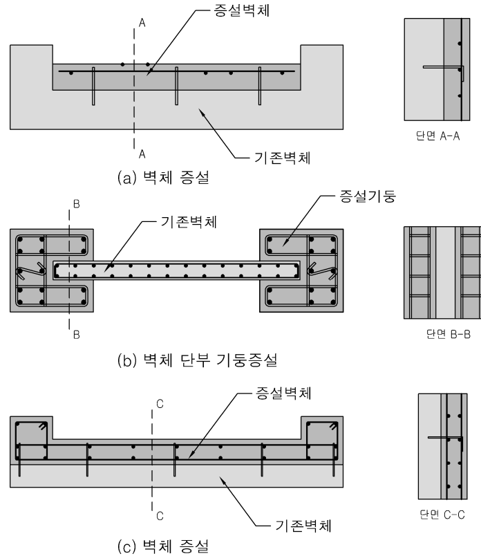
[그림 11-3] 전단벽의 증설
