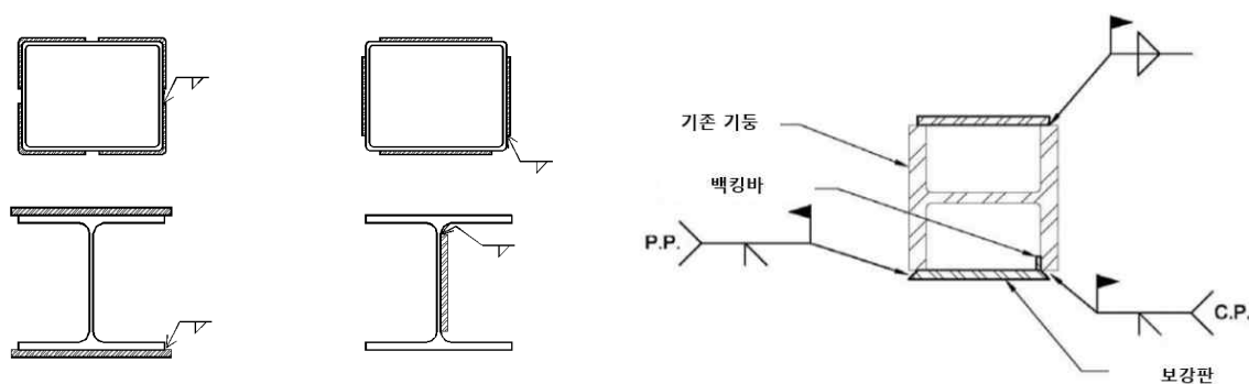
[그림 14-1] 기둥 단면 보강 사례
