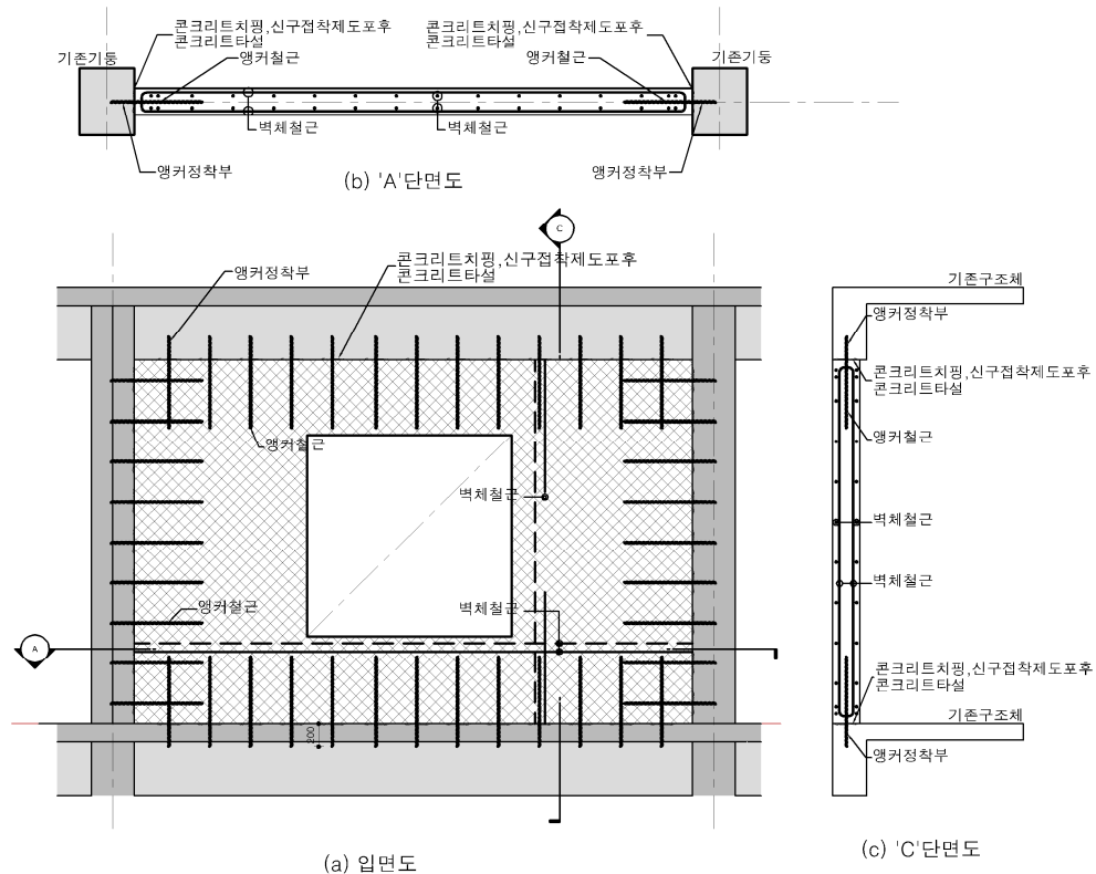
[해그림 11-1] 전단벽에 의한 보강상세
