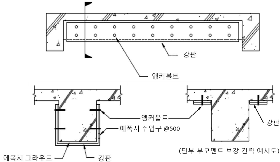
[그림 12-6] 보 강판 보강 공법
