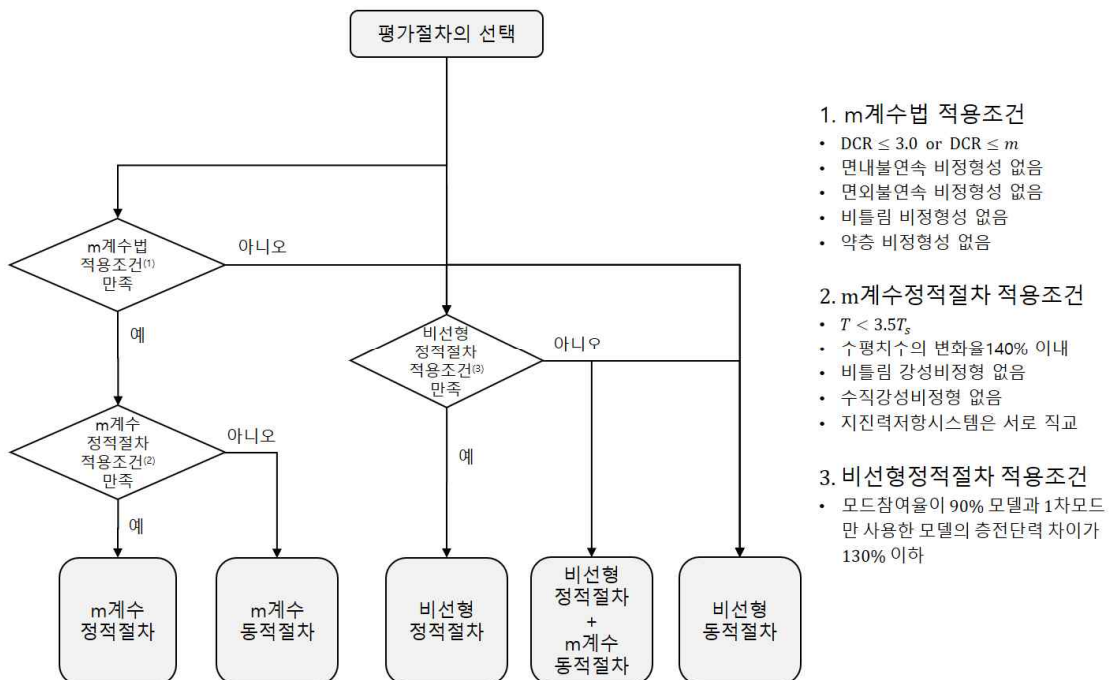
[해그림 4-5] m 계수법, 비선형정적절차, 비선형동적절차 선택을 위한 조건
